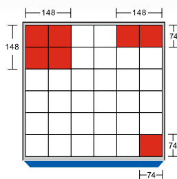
EA型抽屉
